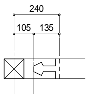
土台の継手寸法図 A2:1/20 A3:1/28
